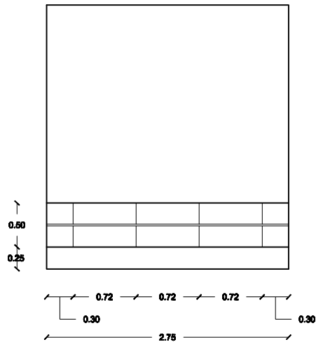
ALZADO
