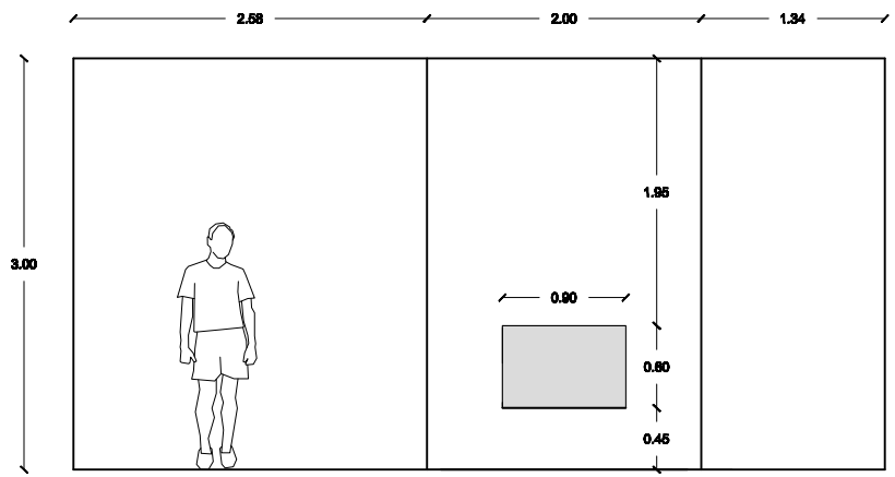
ALZADO CHIMENEA
