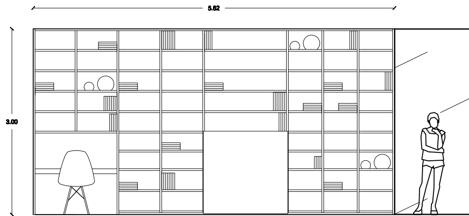
ALZADO MUEBLE SALÓN
