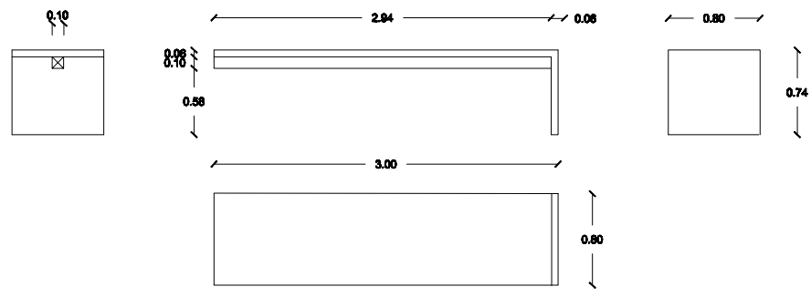
DETALLE MESA DE COMEDOR
