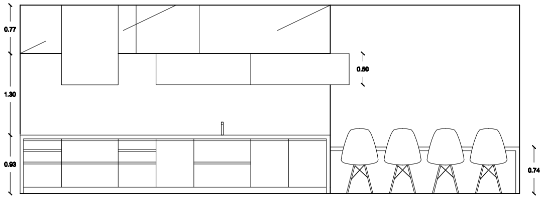
ALZADO COCINA
